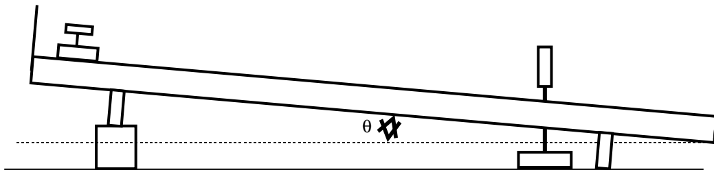
Fig. 1 – Representação esquemática do arranjo experimental para o trilho inclinado.
